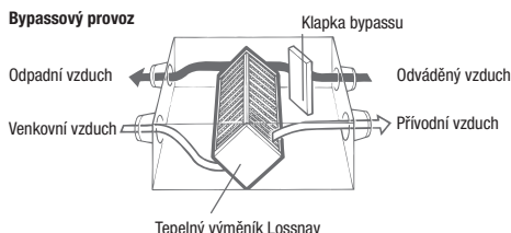
Bypassový provoz
