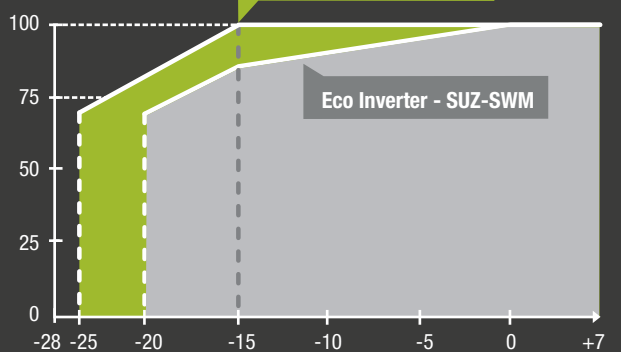
Graf závislosti výkonu od vonkajšej teploty
